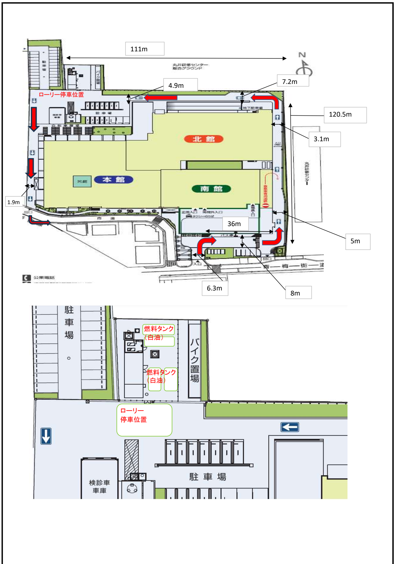
タンク配置図(構内図)
